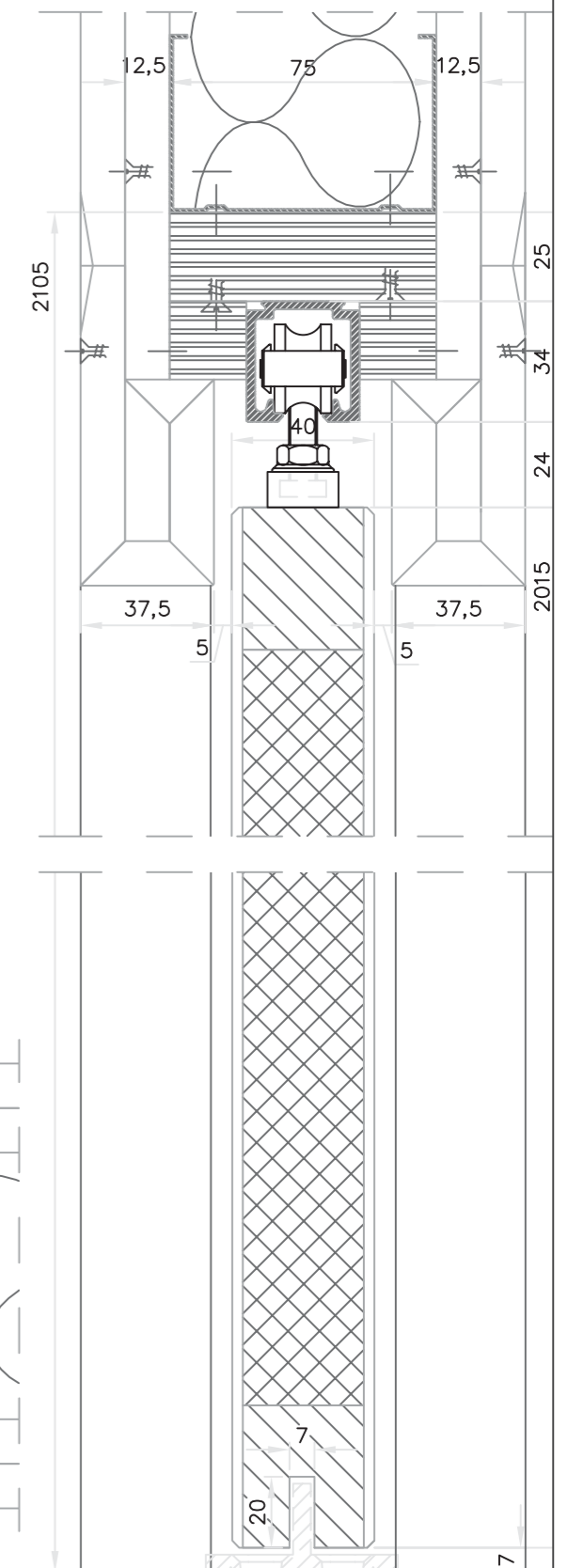
Vertikální řez
