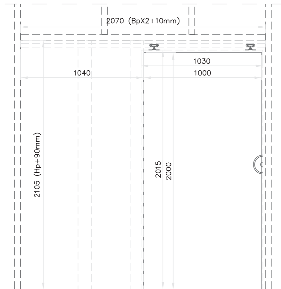
Čelní pohled
