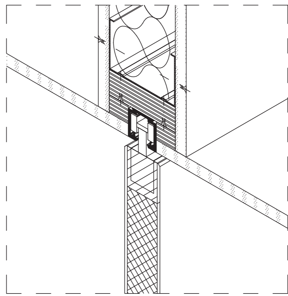
Montážní instrukce
