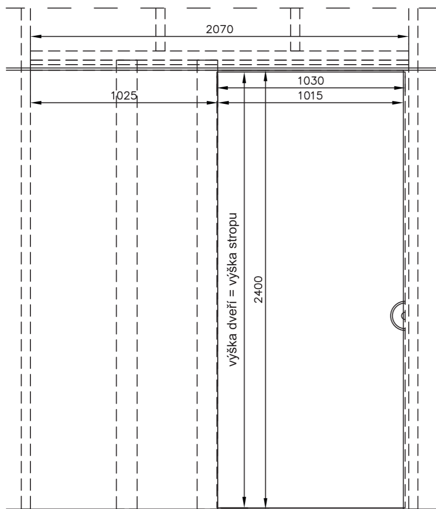
Čelní pohled
