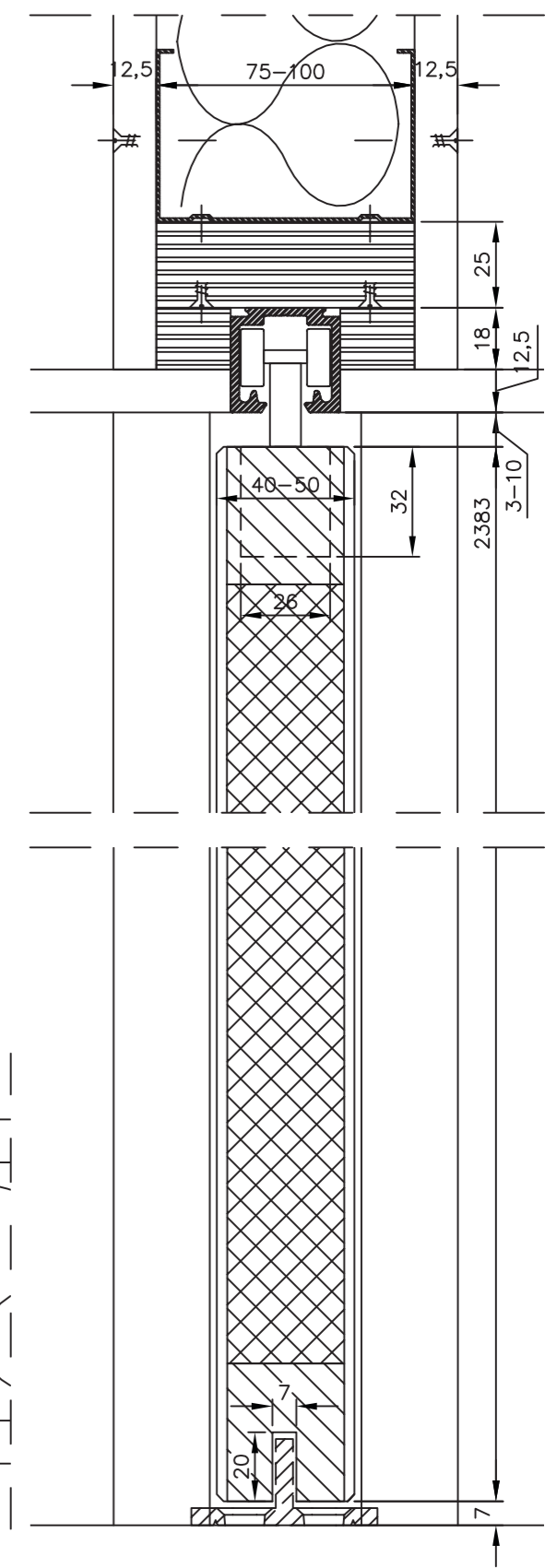
Vertikální řez
