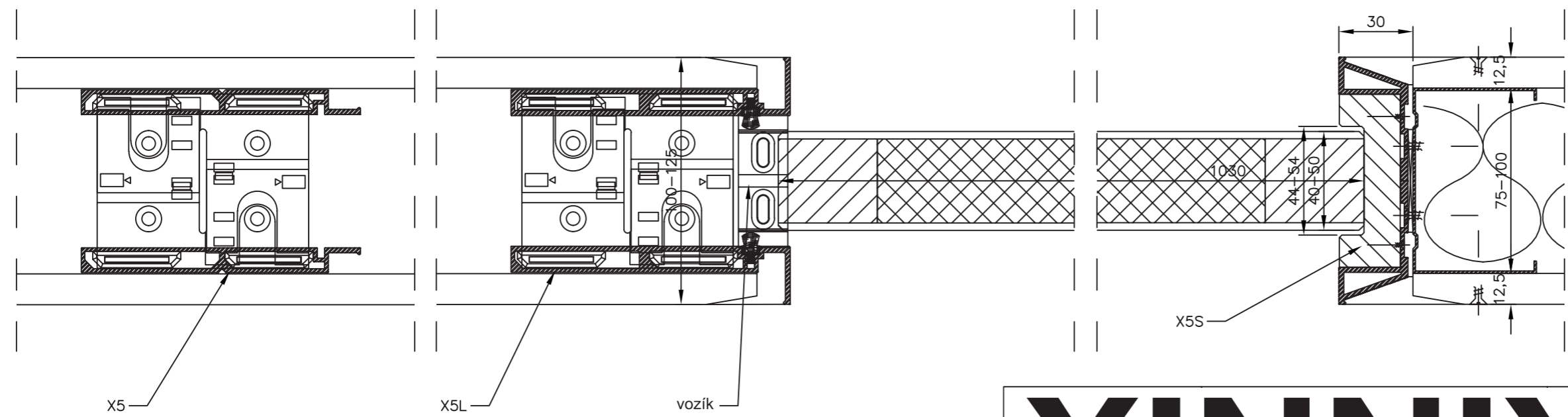
Horizontální řez
